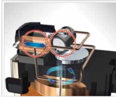
Обычный компрессор
